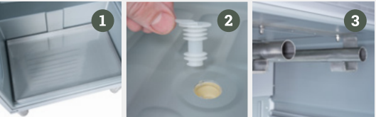
1 Edelstahl-Schweißwanne inklusive 2 Reinigungsablauf mit Schlauchanschluss (unten) 3 Flex-Wildgehänge serienmäßig
